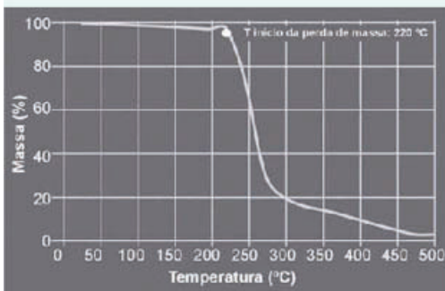
Análise termogravimétrica
